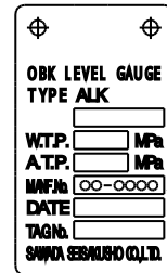
銘板図
