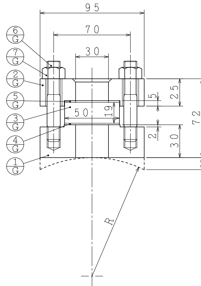
断面 A-A'
