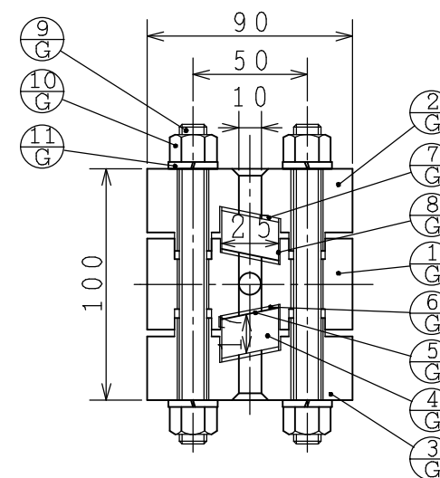
断面 A-A'
